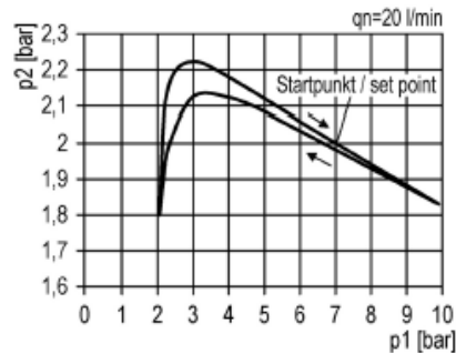
Hysterese
