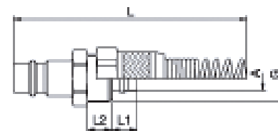
Nippel für Schlauch mit Überwurfmutter und Knickschutzfeder
